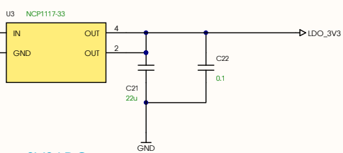
3V3 LDO
